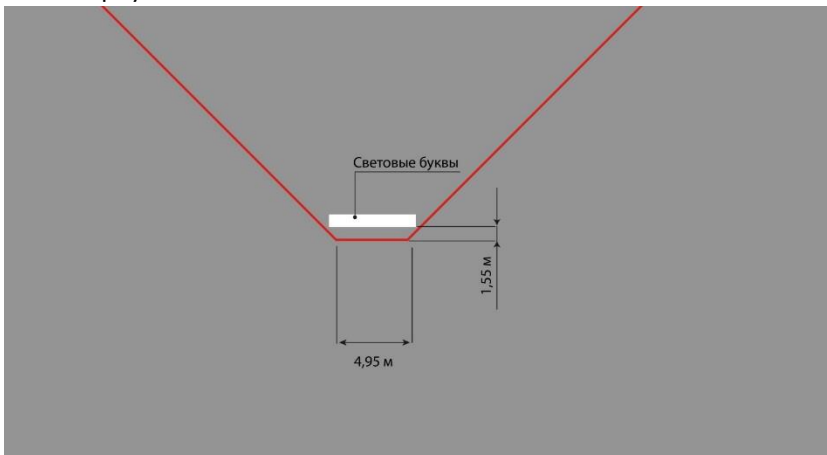
Вид сверху
